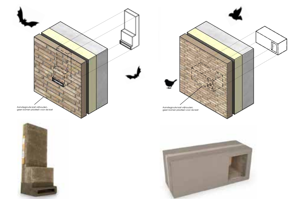
vleermuiskast integreren in gevel mussen-/mezen-/etc-kast integreren in gevel
